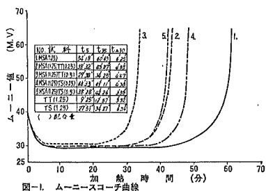
図-1. ムーニースコーチ曲線
