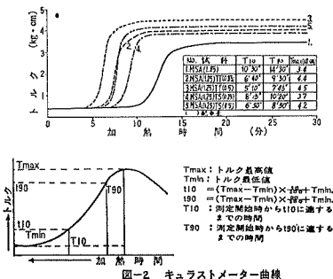
図-2. キュラストメーター曲線
