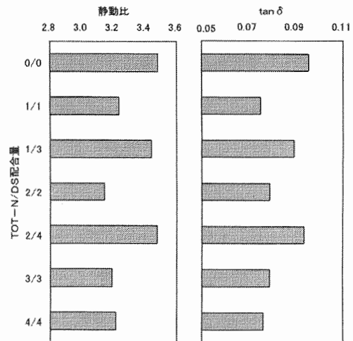
図1 TOT-N/助剤DS配合量と防振ゴム特性
