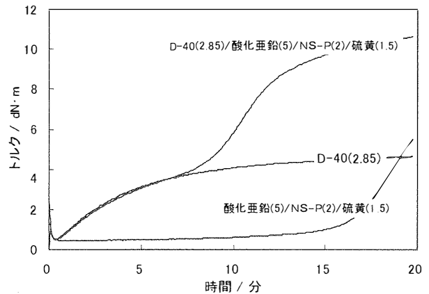
図2 過酸化化物加硫と硫黄加硫(NS-P)の併用
