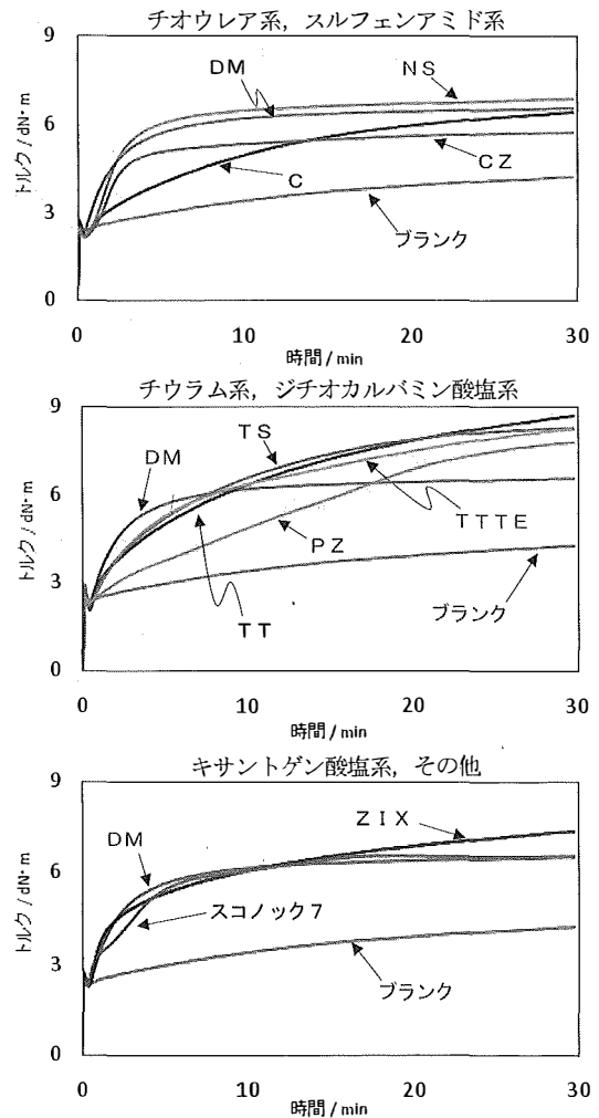
図1 加硫試験結果
