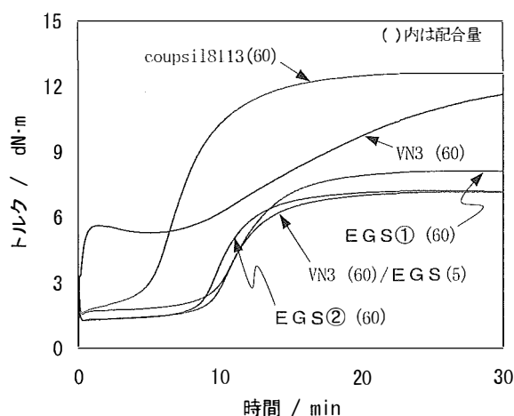
図1 加硫曲線(測定温度160℃)
