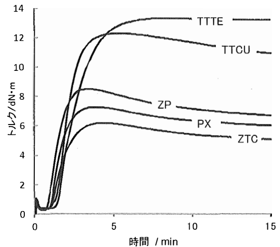
図2 ジチオカルバミン酸塩系加硫促進剤の加硫曲線②
