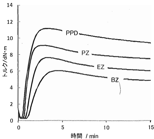
図1 ジチオカルバミン酸塩系加硫促進剤の加硫曲線●
