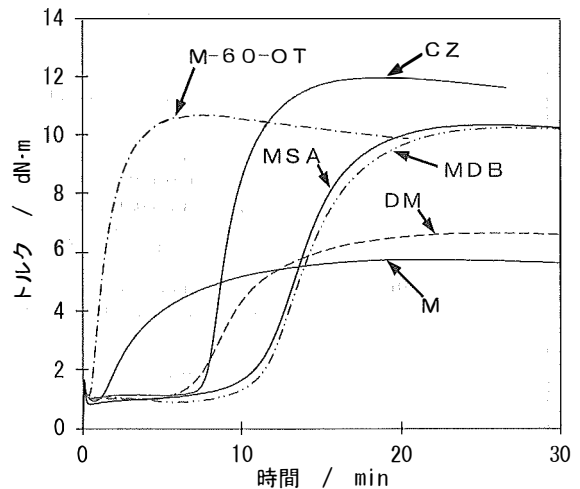
図2 チアゾール系、スルフェンアミド系の加硫曲線
