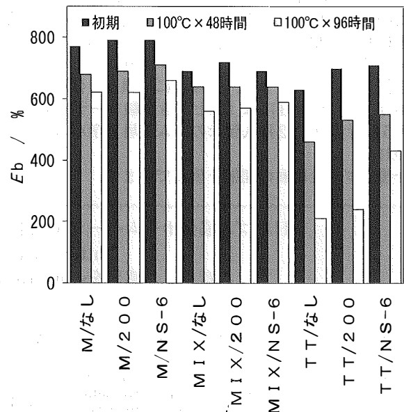
図2 初期と熱老化後の E_b
