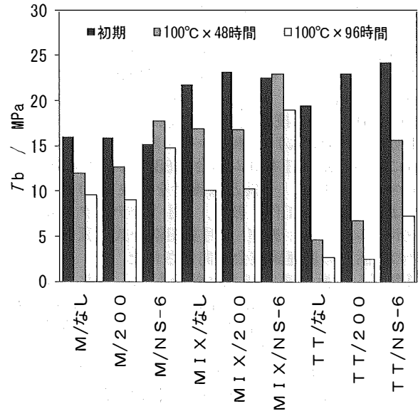
図1 初期と熱老化後の T_b
