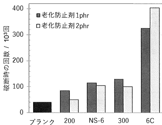
図2 100℃での破断時の回数の中央値
