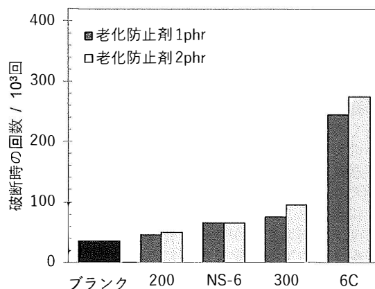
図1 室温での破断時の回数の中央値
