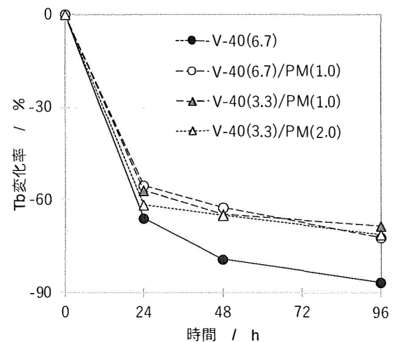
(2) 加硫時間; tc(90) × 2 図1 熱老化時間とTb変化率
